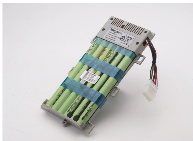
Una batería de iones de litio ligera de alta potencia reemplazable por el usuario permite realizar, con una sola carga, 200 pruebas de 100 A manuales/automáticas o hasta dos pruebas de 100 A en modo continuo de 10 minutos de duración; cuando se encuentra completamente vacía, tarda dos horas y media en cargarse.
