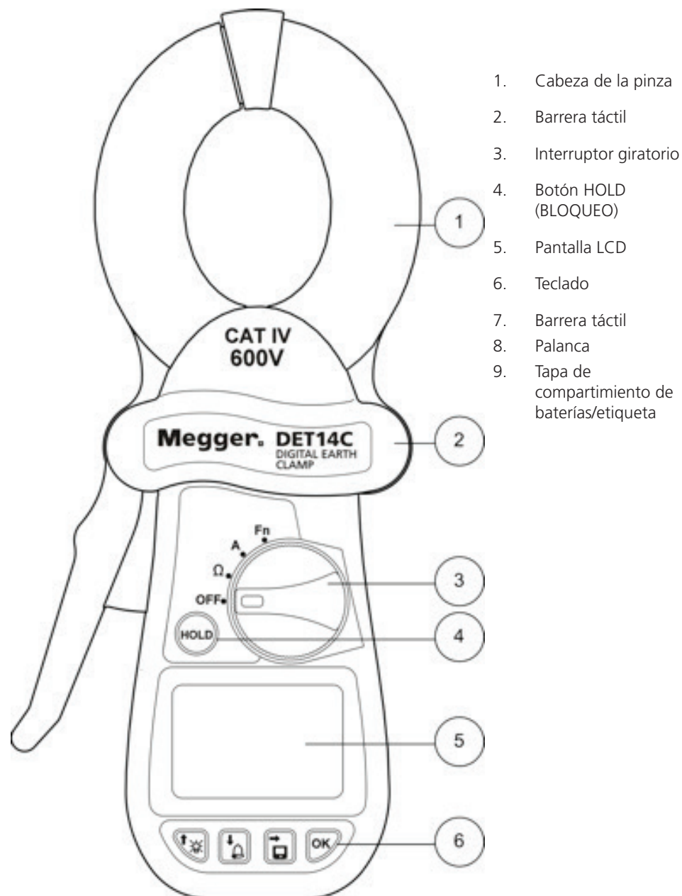
Figura 1: DET14C / DET24C Vista frontal del instrumento
